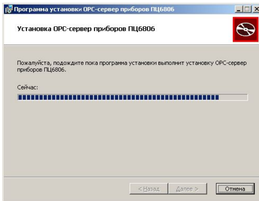
Рисунок 3.5 - Копирование файлов
