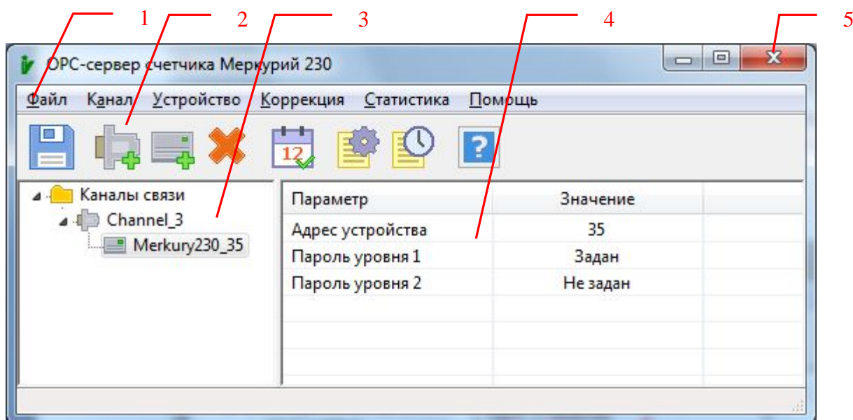
Рисунок 6.1 - Окно конфигурации ОПС-сервера
