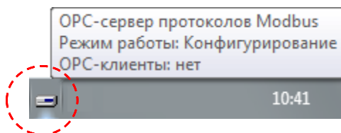
Рисунок 6.3 – Значок в области уведомлений Windows
