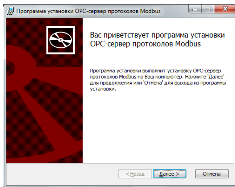
Рисунок 3.1 - Окно инсталлятора
