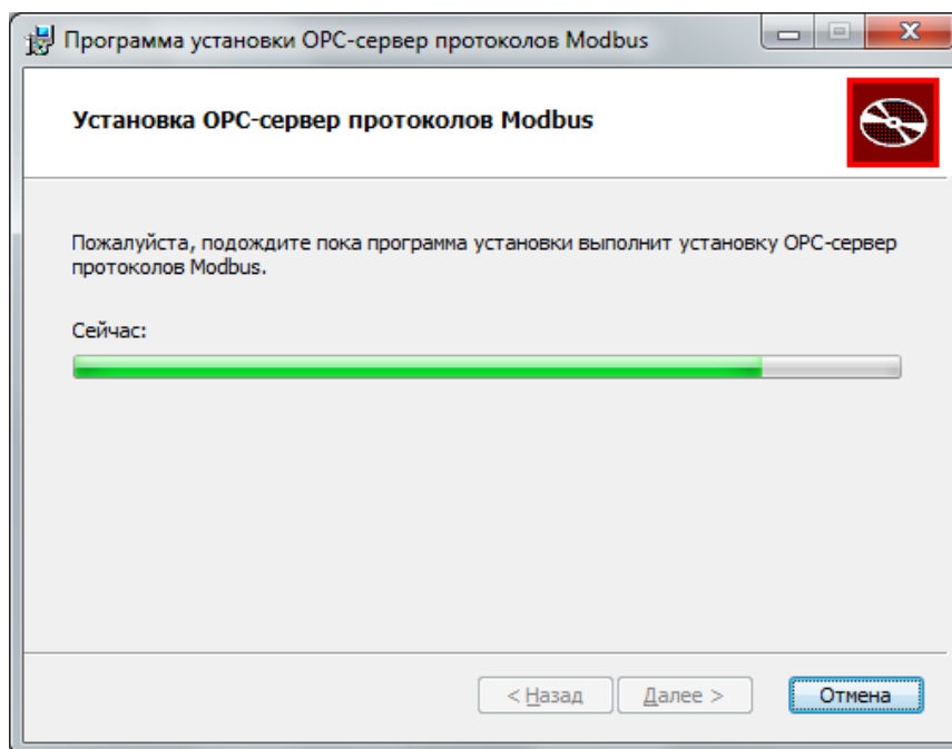
Рисунок 3.5 - Копирование файлов
