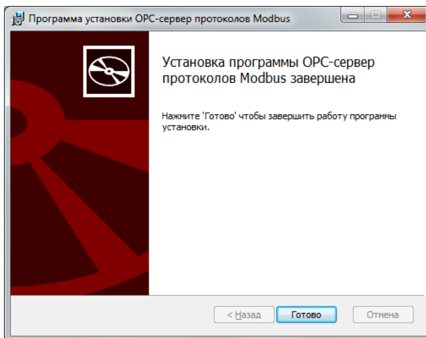
Рисунок 3.6 - Установка завершена
