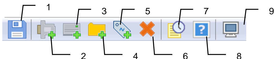
Рисунок 6.2 – Панель инструментов
